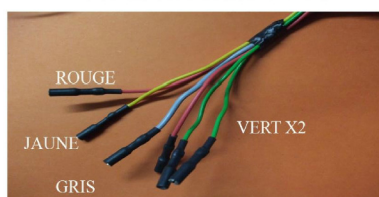
LIAISON FAISCEAU AR
