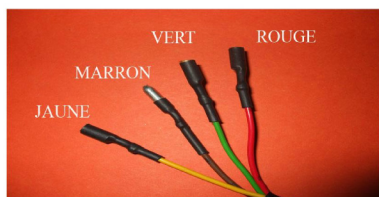
MANO CONTACT HUILE
